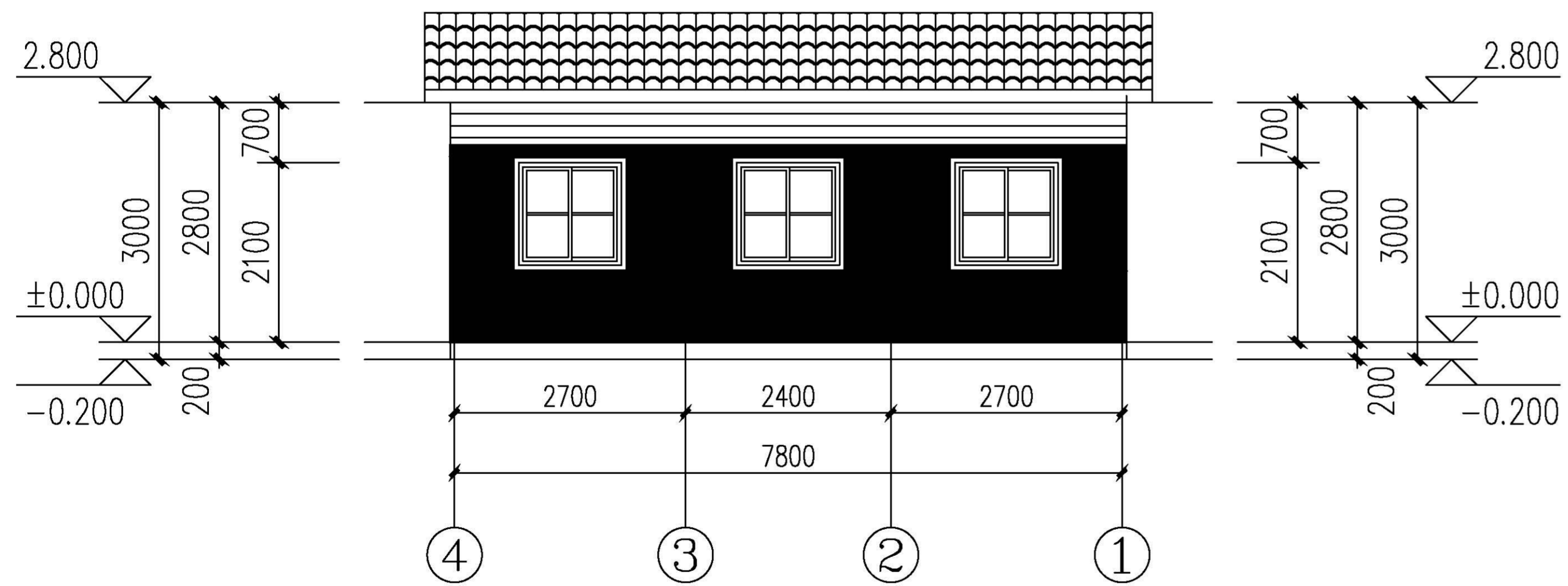
④ ~ ① Elevation 1:100
