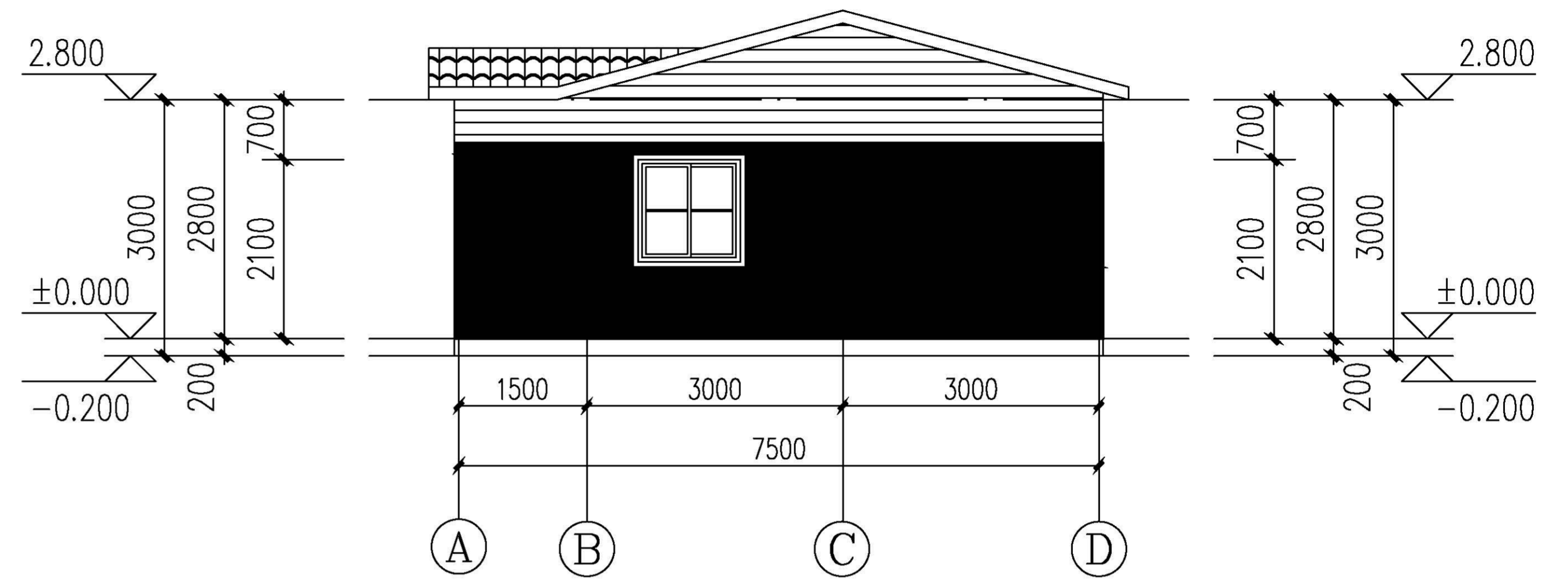
Ⓐ ~ Ⓓ Elevation 1:100
