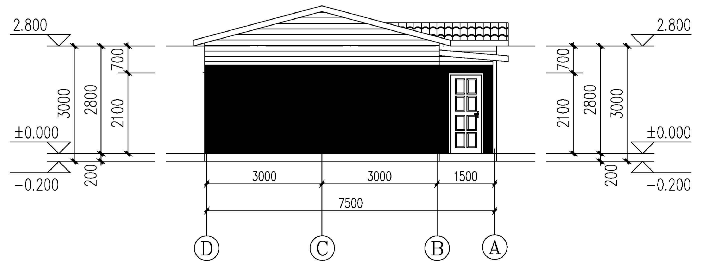
Ⓓ ~ Ⓐ Elevation 1:100
