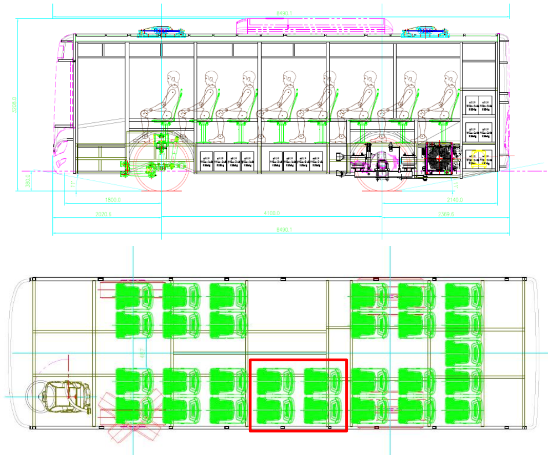
车辆布置图 Bus Layout
