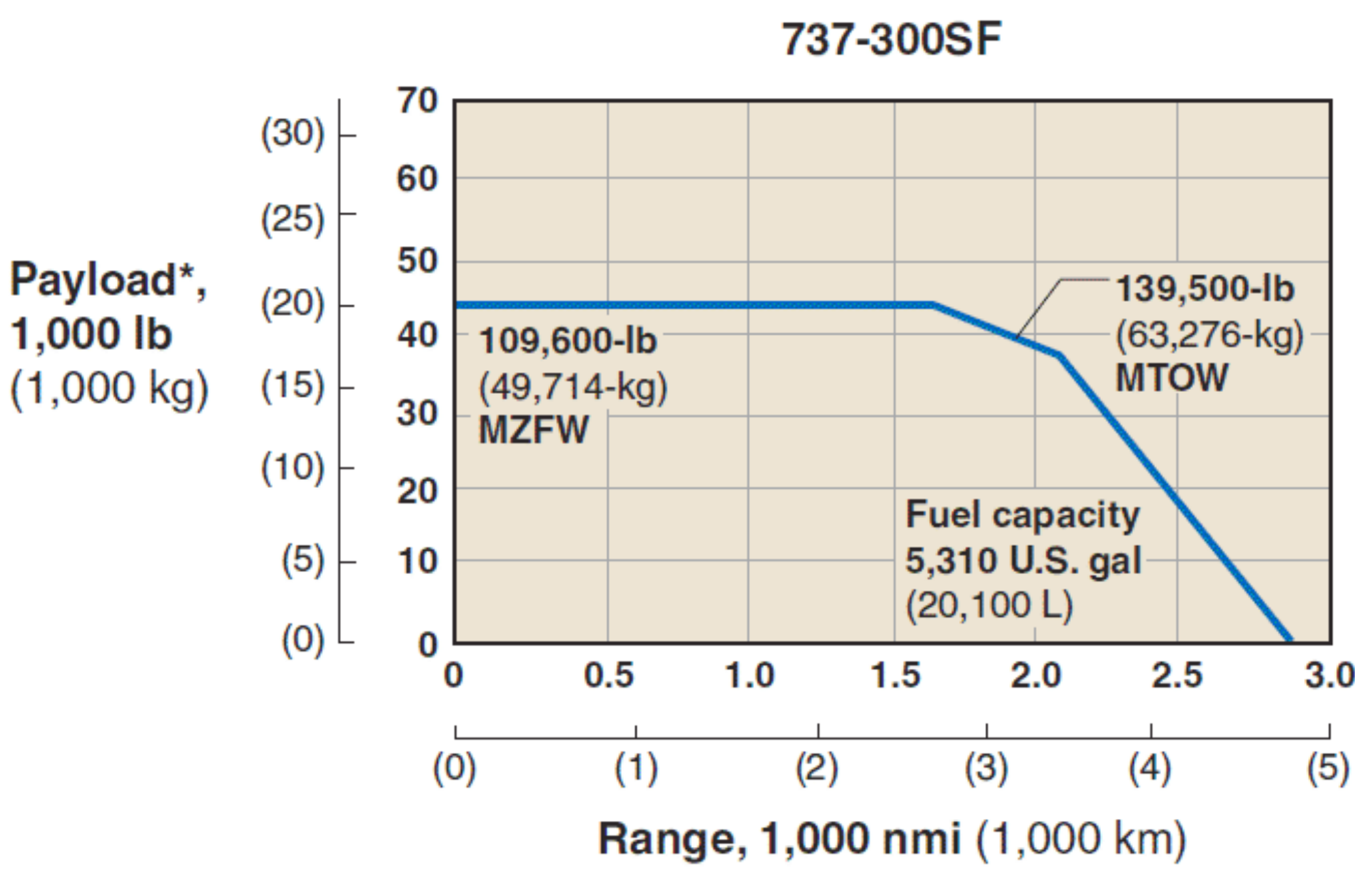
Payload-Range
