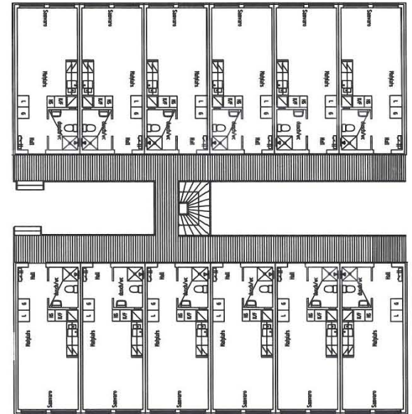
BOTTENVÄNING
